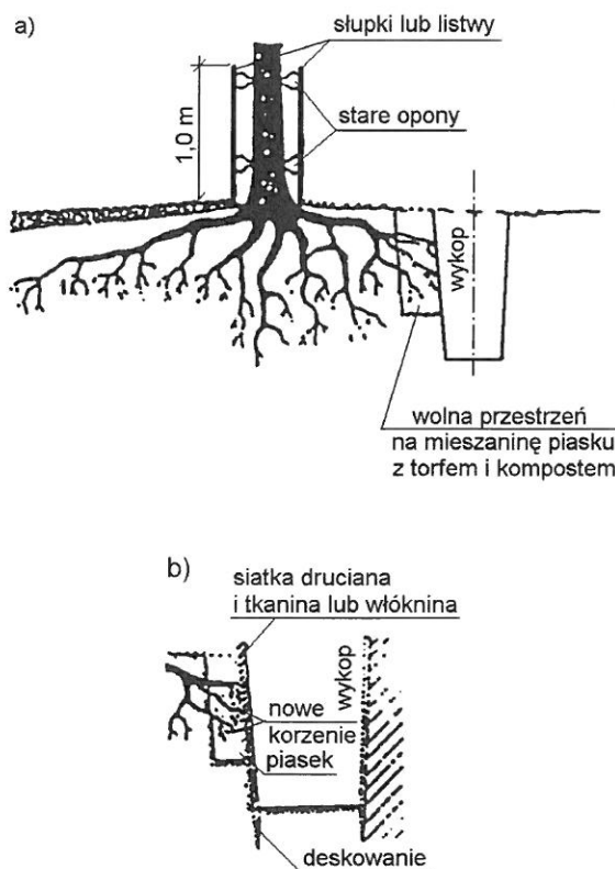
Rys. 1. Wykonywanie wykopów instalacyjnych w obrębie strefy korzeniowej drzew
